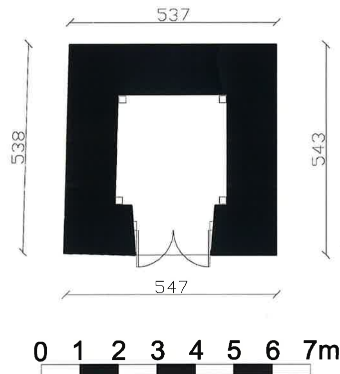
RZUT PRZYZIEMIA skala 1:100
